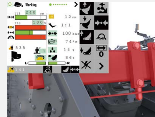
Senzorul de pe cadrul principal măsoară presiunea de compactare aplicată. Valorile măsurate sunt afișate pentru operator pe CEMIS 700. Sistemul reglează limitele de încărcare pe baza acestor valori.
